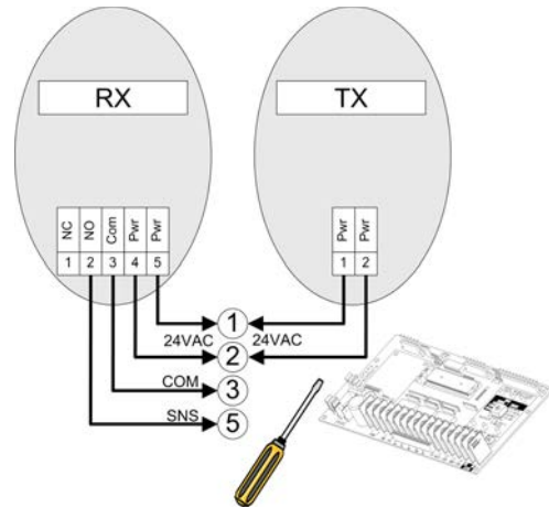
Figure 18 - PHOTO 015 / 016 / 045 / 050 / 051 / 059
